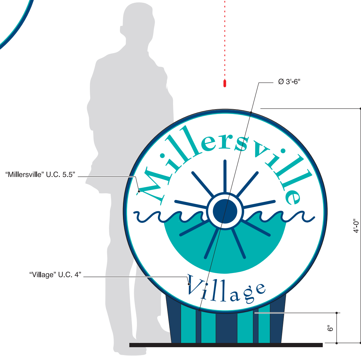
1 Elevation - Faces A/B scale: 1"=1'-0"
